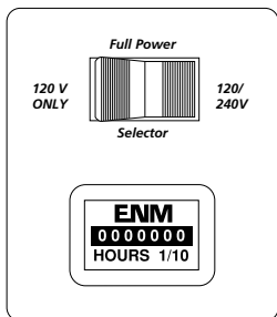
120/240 VOLT Position
